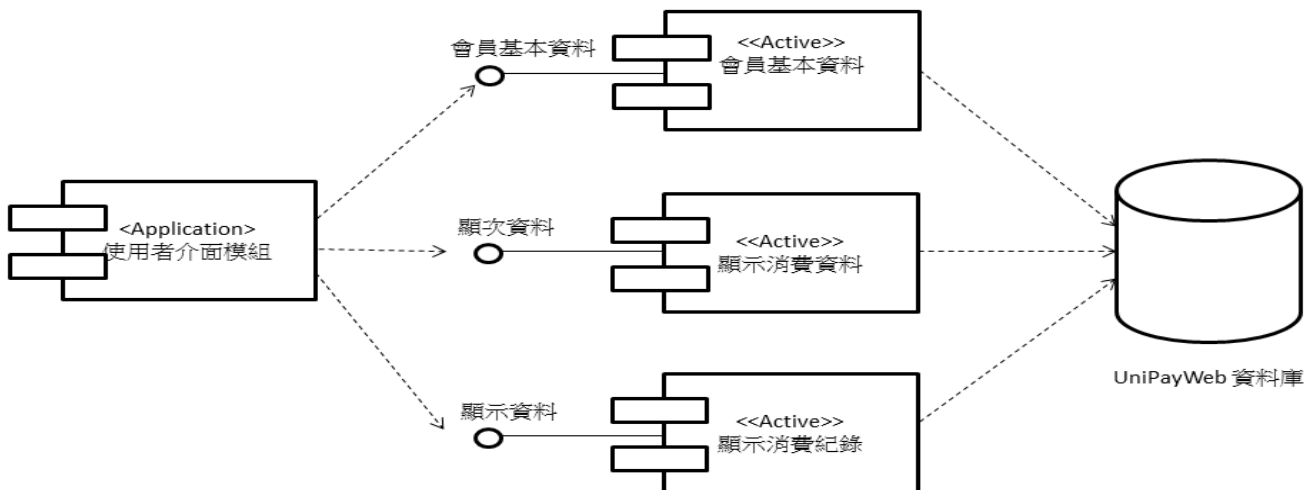
一般會員元件圖
