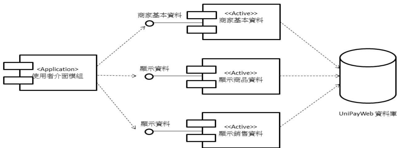
一般商家元件圖
